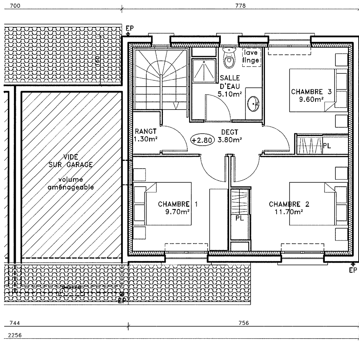
ETAGE SURFACE HABITABLE : 41.20m 2
