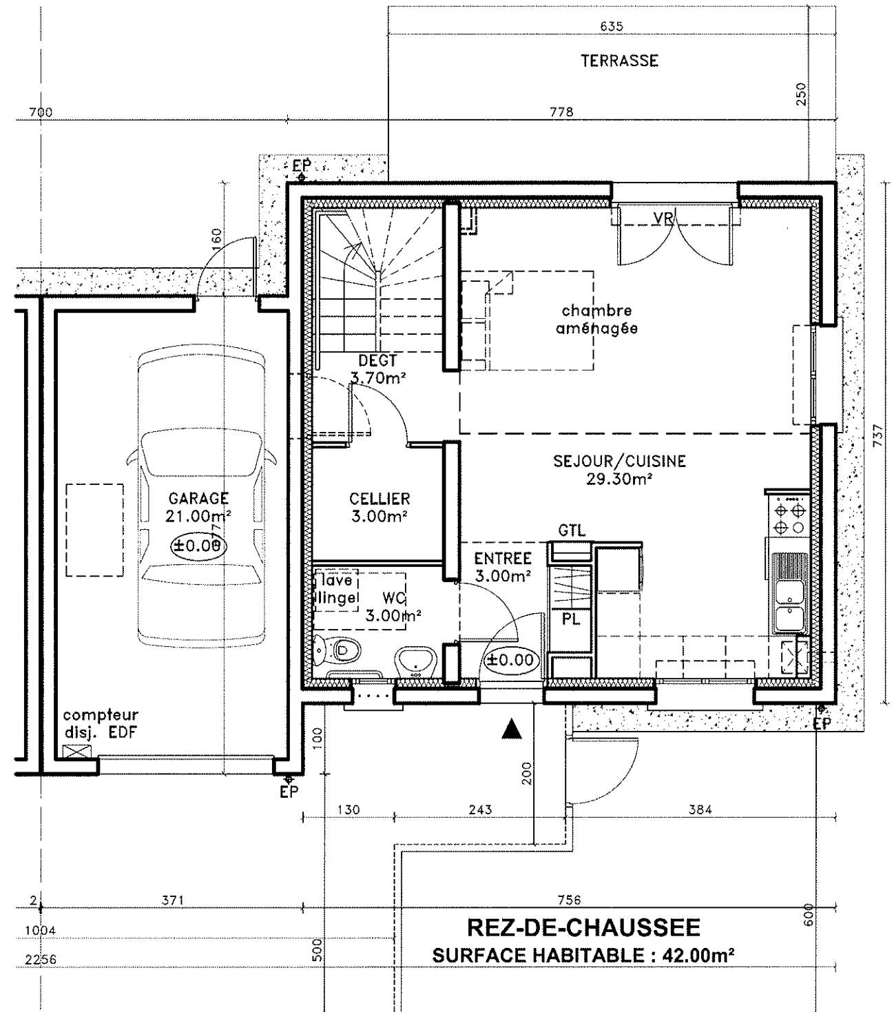
PLAN LOGEMENT TYPE T4a SURFACE HABITABLE TOTALE : 83.20m 2 Echelle 1/100 15 décembre 2011
